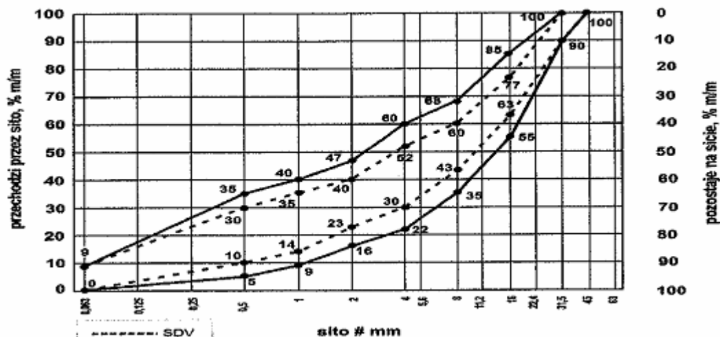
Rysunek 1. Pole dobrego uziarnienia kruszywa przeznaczonych na podbudowę wykonywane metodą stabilizacji mechanicznej 0/31,5
