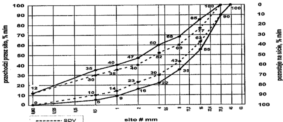
Rys. nr 2 Krzywa uziarnienia – mieszanka niezwiązana 0/31,5 do warstwy podbudowy pomocniczej KR3
