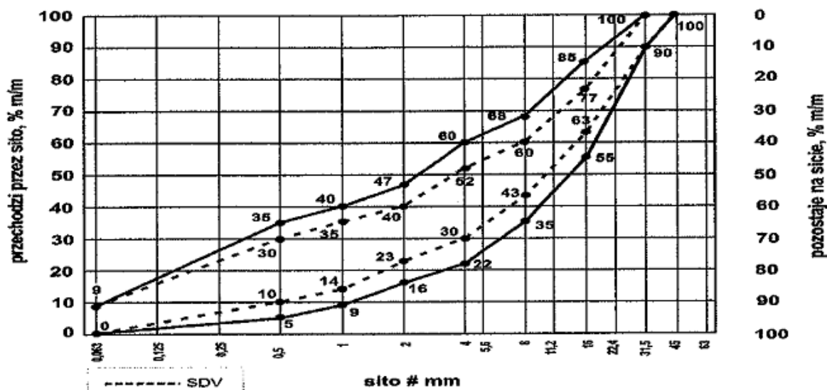
Rys. nr 1. Krzywa uziarnienia – mieszanka niezwiązana 0/31,5 do dla warstwy podbudowy zasadniczej KR 2
